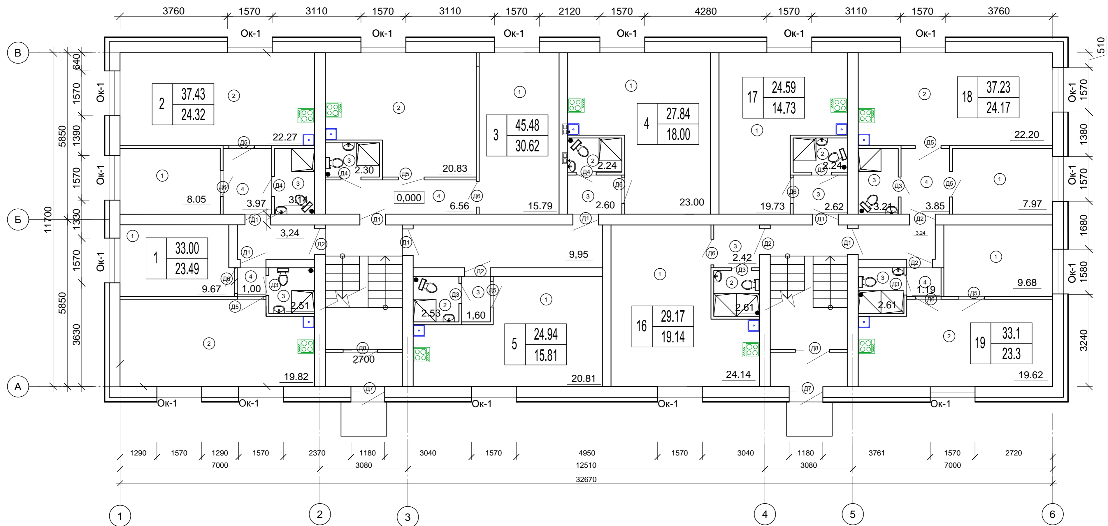
Экспликация помещений
